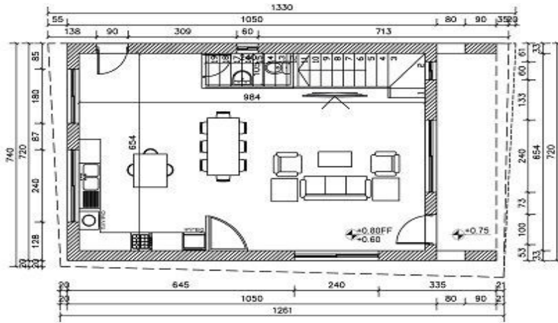
ΚΑΤΟΙΚΙΑ 5 ΚΑΤΟΨΗ ΙΣΟΓΕΙΟΥ
