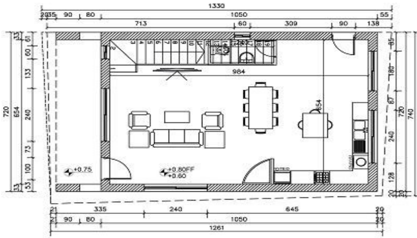
ΚΑΤΟΙΚΙΑ 6 ΚΑΤΟΨΗ ΙΣΟΓΕΙΟΥ
