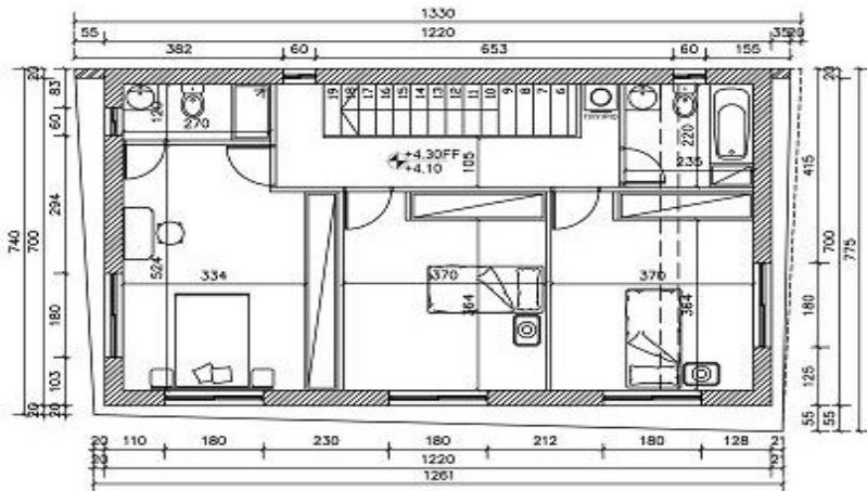
ΚΑΤΟΙΚΙΑ 5 ΚΑΤΟΨΗ ΟΡΟΦΟΥ
