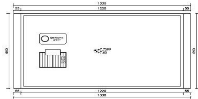
ΚΑΤΟΙΚΙΑ 1 ΚΑΤΟΨΗ ΟΡΟΦΗΣ
