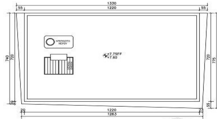
ΚΑΤΟΙΚΙΑ 5 ΚΑΤΟΨΗ ΟΡΟΦΗΣ
