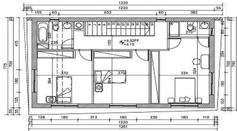
ΚΑΤΟΙΚΙΑ 6 ΚΑΤΟΨΗ ΟΡΟΦΟΥ
