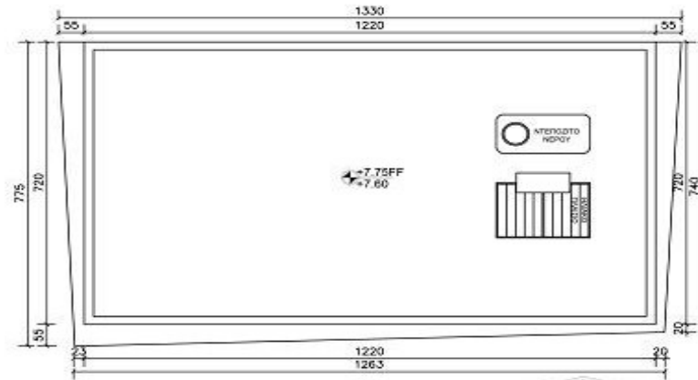
ΚΑΤΟΙΚΙΑ 6 ΚΑΤΟΨΗ ΟΡΟΦΗΣ
